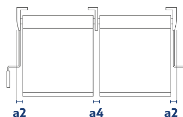
Doble caída 2 accionamientos
